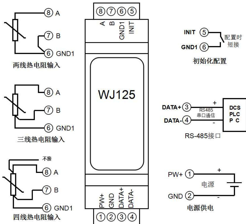
图3 WJ125 模块接线图
