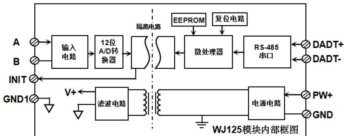
图2 WJ125 模块内部框图
