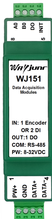
图1 WJ151 模块外观图
