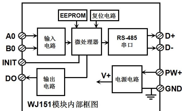
图2 WJ151 模块内部框图
