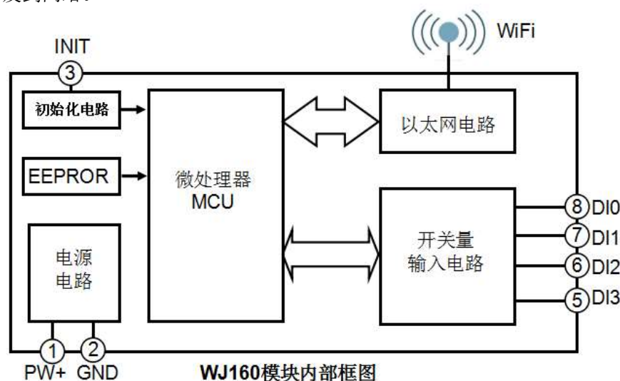
图2 WJ160 模块内部框图
