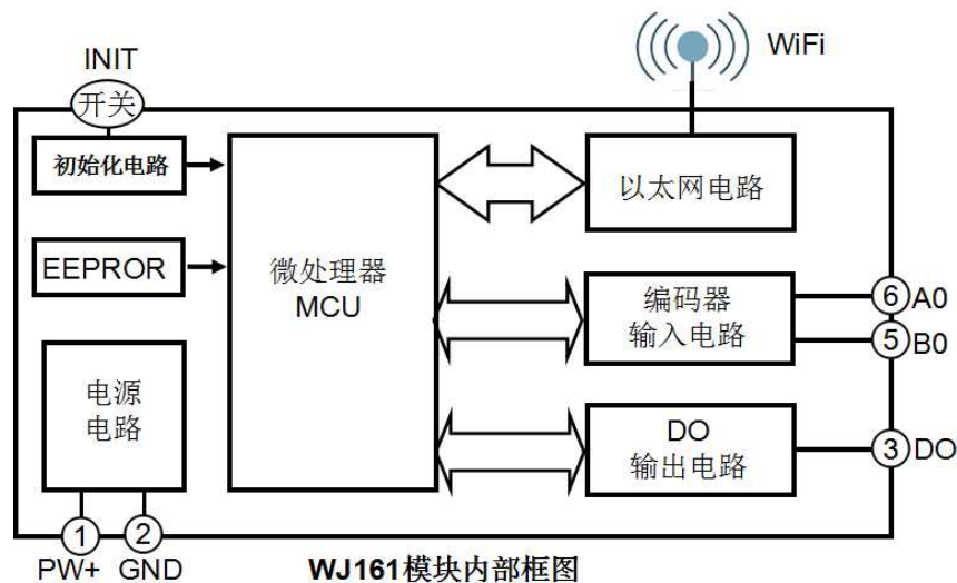
图 2 WJ161P 模块内部框图
