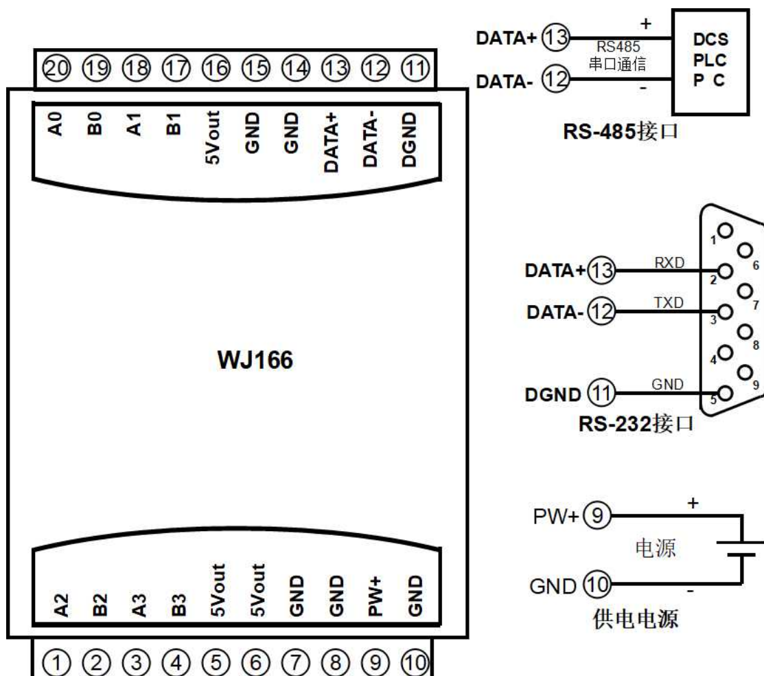
图3 WJ166 模块接线图
