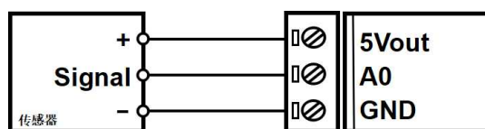
5V 供电的光电开关接线图
