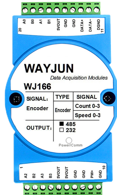
图1 WJ166 模块外观图
