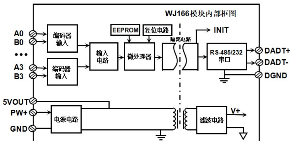
图2 WJ166 模块内部框图
