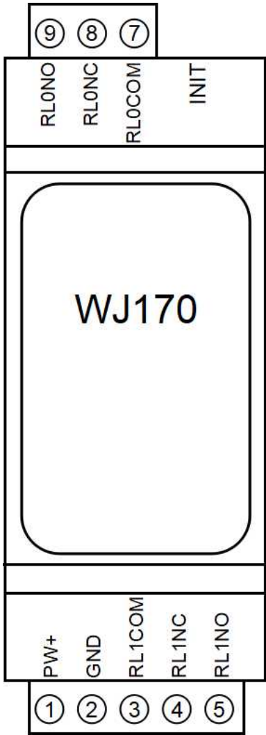
图 3 WJ170 模块接线图
