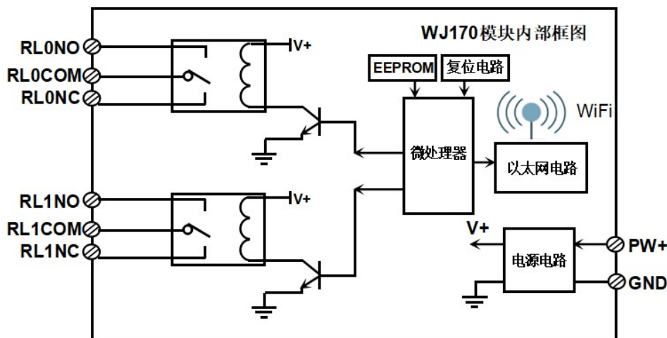
图 2 WJ170 模块内部框图
