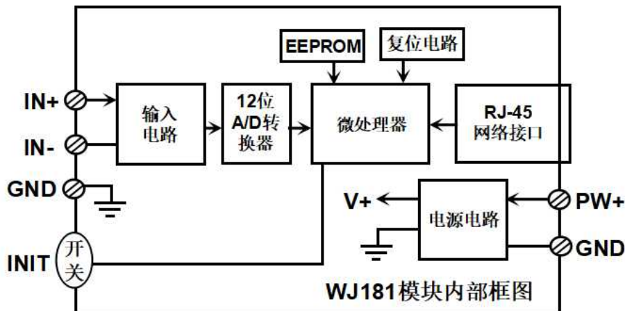
图2 WJ181 模块内部框图
