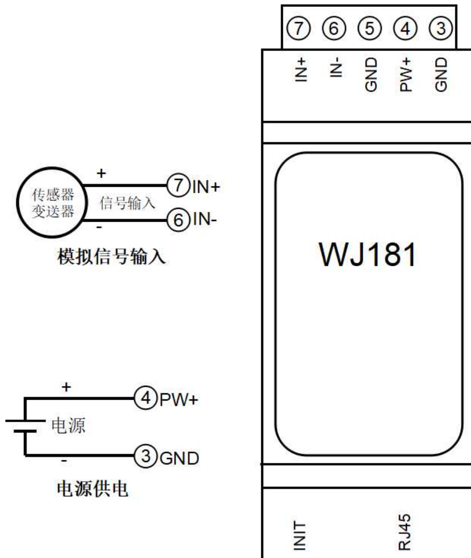
图 3 WJ181 模块接线图
