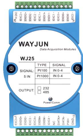
图1 WJ25 模块外观图
