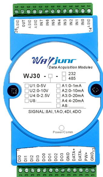
图1 WJ30 模块外观图
