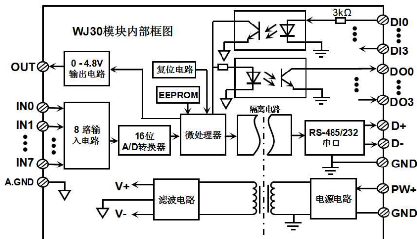
图2 WJ30 模块内部框图
