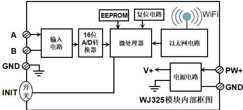
图 2 WJ325 模块内部框图
