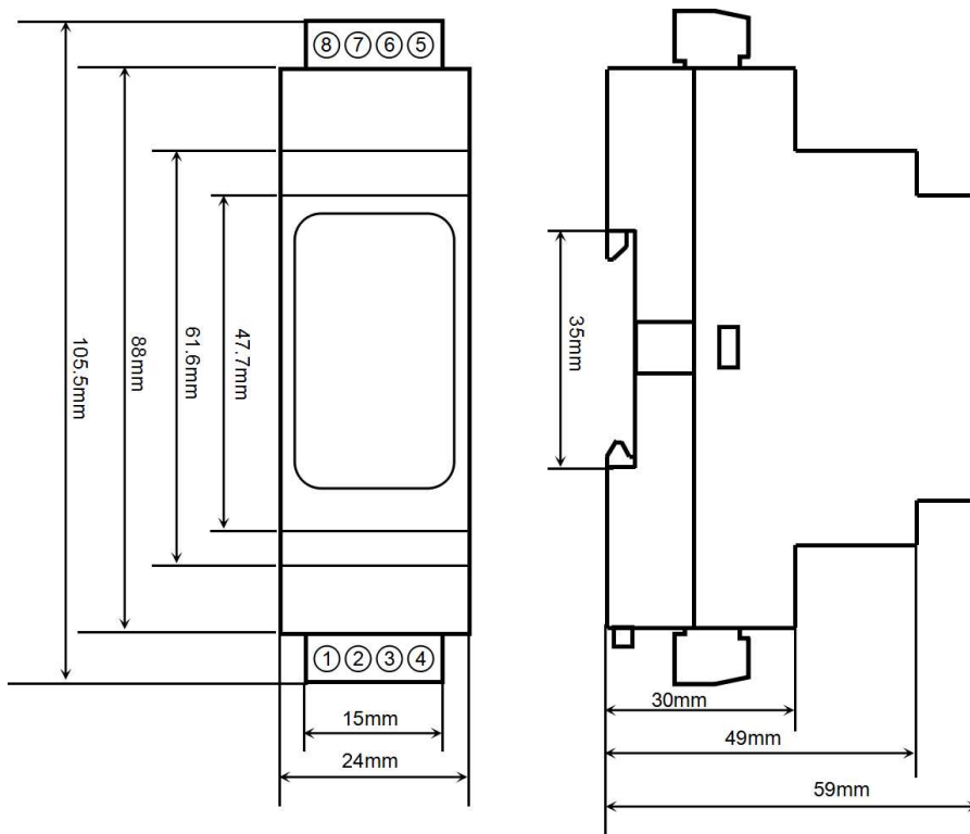
可以安装在标准 DIN35 导轨上
