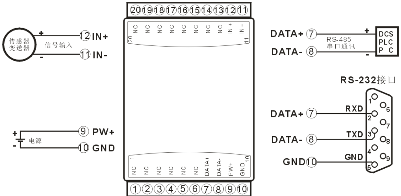
图3 WJ63 模块接线图
