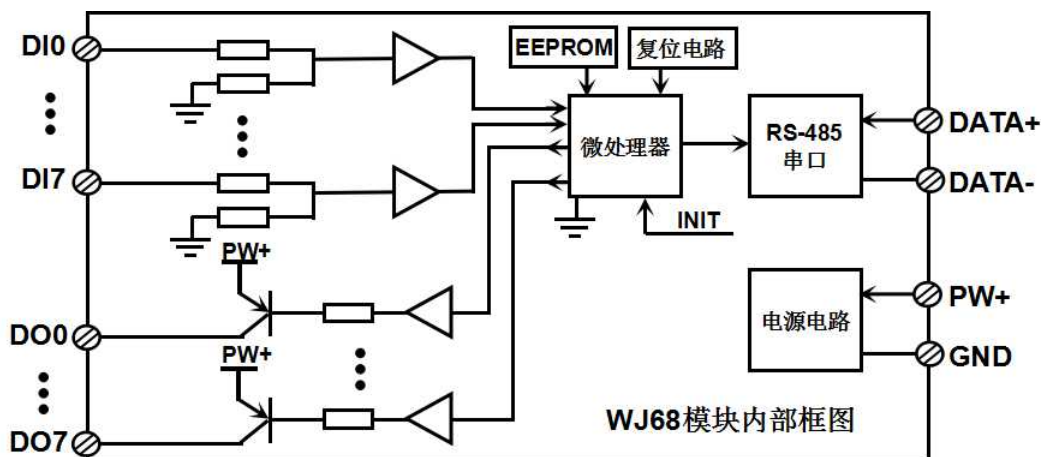
图2 WJ68 模块内部框图
