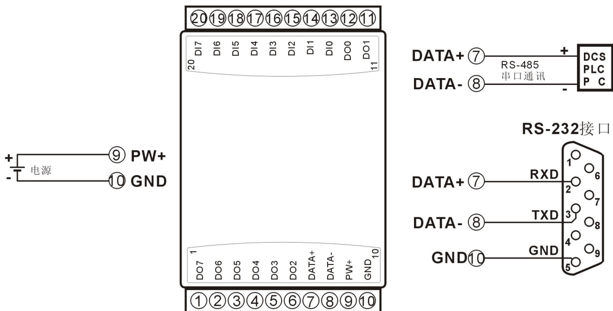
图 3 WJ68 模块接线图
