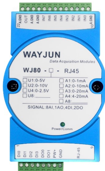
图1 WJ80 模块外观图
