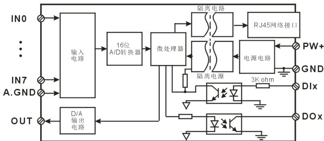
图2 WJ80 模块内部框图
