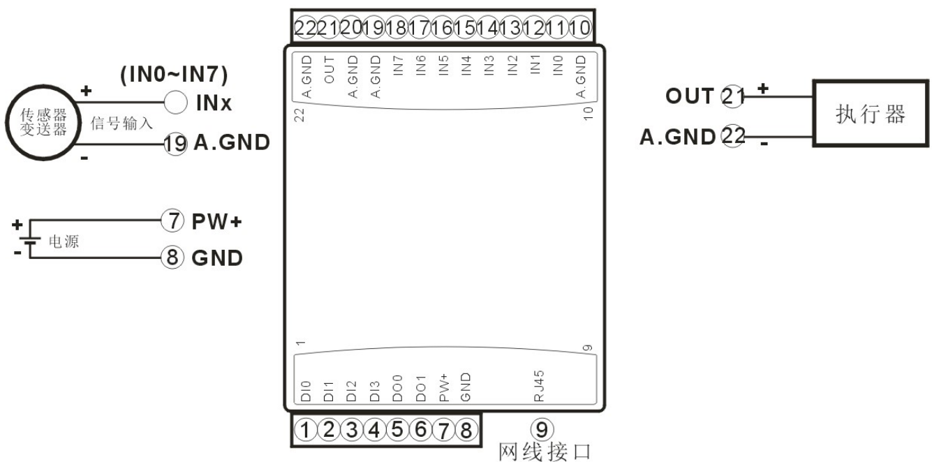
图 5 WJ80 模块接线图
