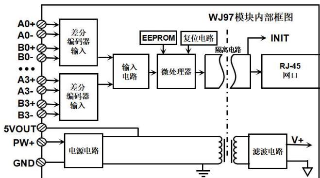
图2 WJ97 模块内部框图
