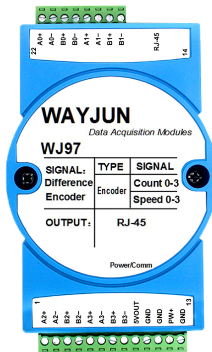
图1 WJ97 模块外观图
