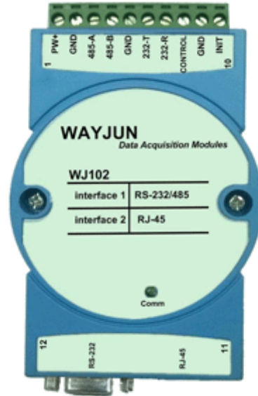
图 1 WJ102 模块外观图
