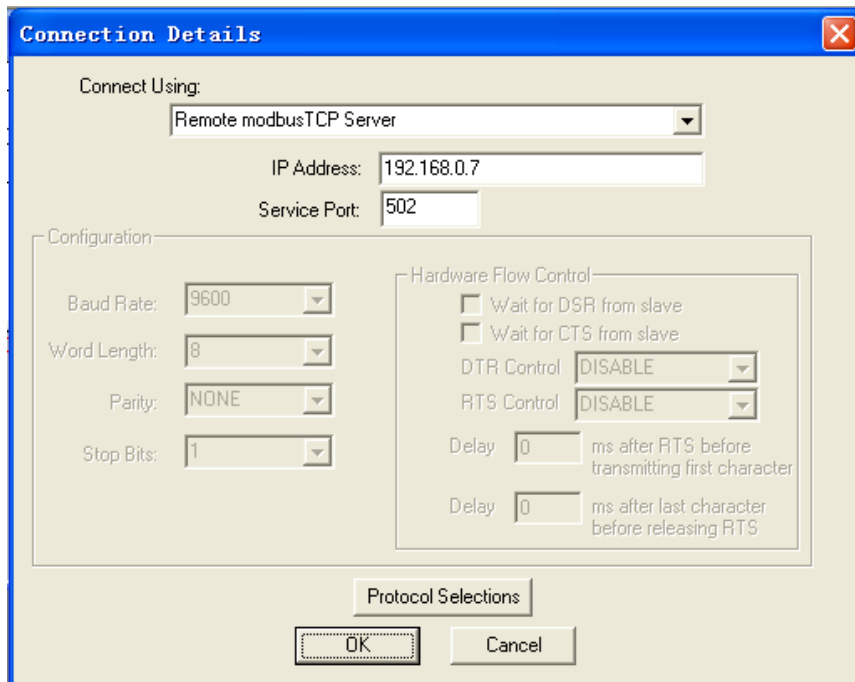
图 5 WJ102 使用 ModScan32 软件 的设置
