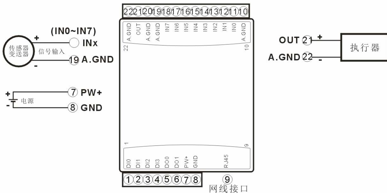
图 5 WJ80 模块接线图
