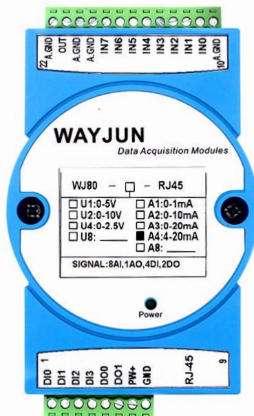
图1 WJ80 模块外观图
